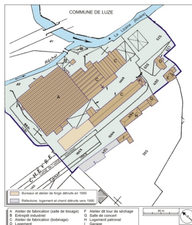
Plan-masse. Extrait du plan cadastral numérisé, 2005, section A, 1:1250. Dess. André Céréza IVR43_20067000042NUDA
