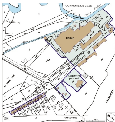
Plan de situation. Extrait du plan cadastral numérisé, 2005, section A, 1:1250 réduit à 1:2000. Dess. André Céréza IVR43_20067000041NUDA
