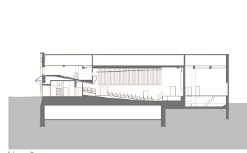
Coupe longitudinale. D'après une coupe de l'atelier Correia Architectes et Associés.
