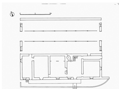
Plan au sol. Phot. Dominique et Sancey Dominguez IVR43_19792500015V
