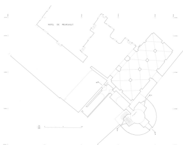
Tour Renard : plan du niveau inférieur. Dess. Alain Morelière IVR26_20122100101A2YY
