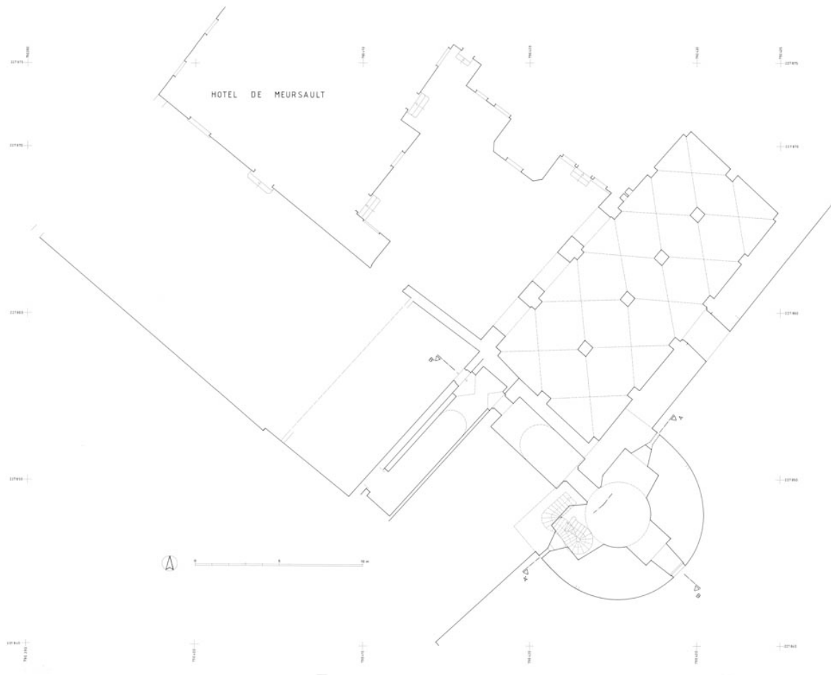
Tour Renard : plan du niveau inférieur.
