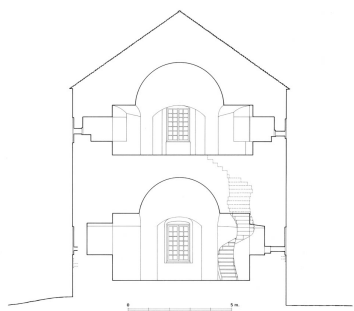
Tour Renard : coupe longitudinale. Dess. Alain Morelière IVR26_20122100103A2YY
