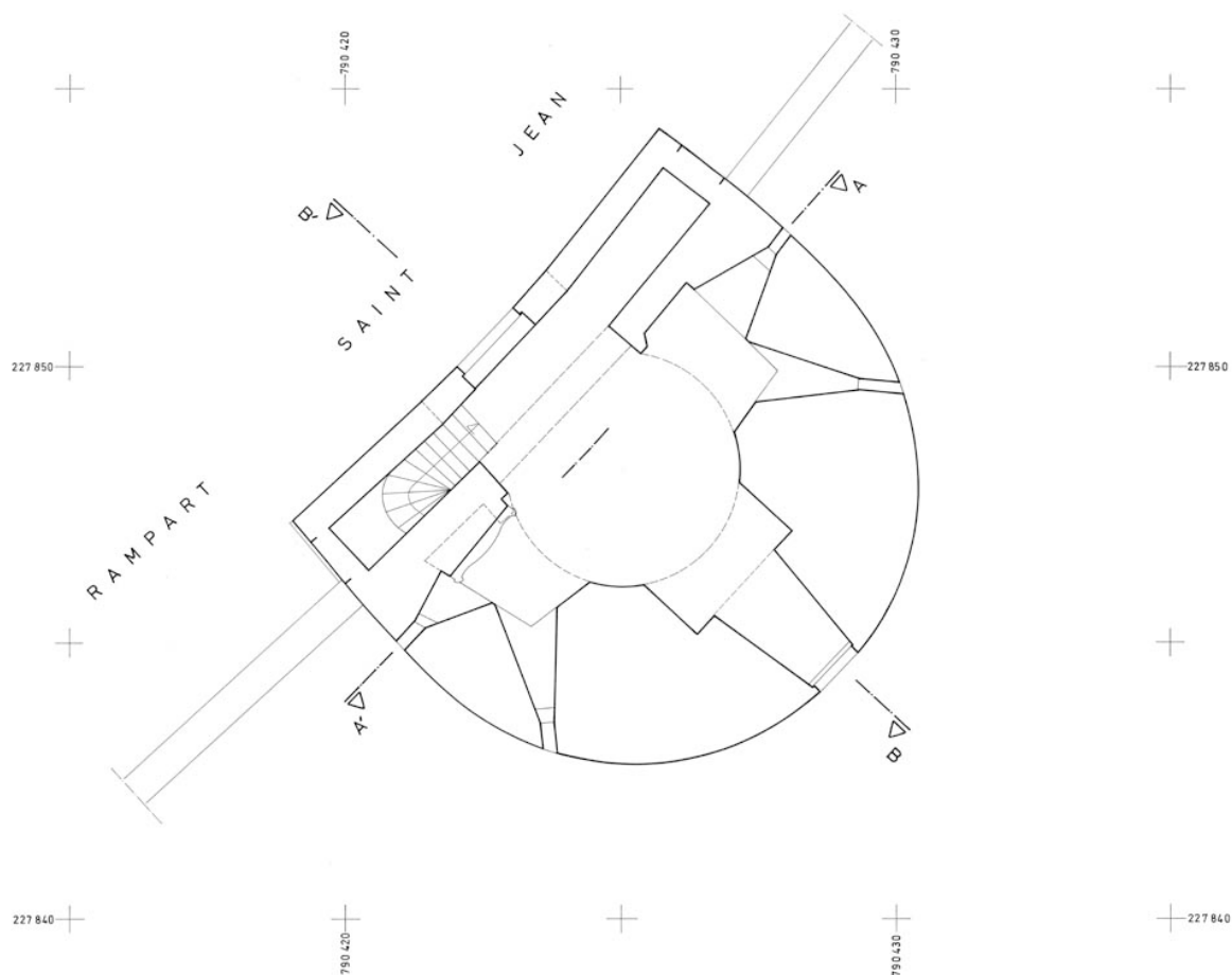
Tour Renard : plan du niveau supérieur.
