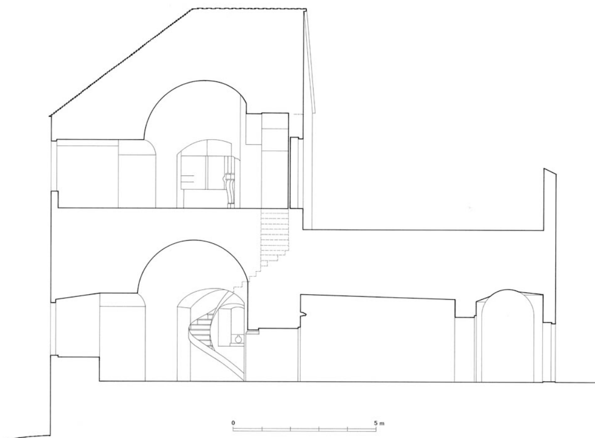
Tour Renard : coupe transversale.
