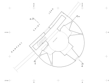
Tour Renard : plan du niveau supérieur. Dess. Alain Morelière IVR26_20122100102A2YY
