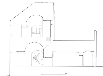
Tour Renard : coupe transversale. Dess. Alain Morelière IVR26_20122100104A2YY
