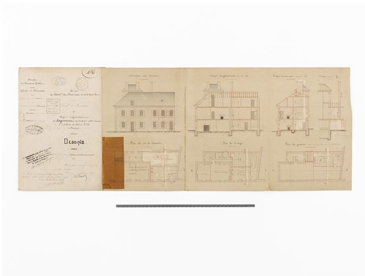
"Projet d'agrandissement du Logement du Conducteur subdivisionnaire à l'Ecluse de Loire n°35 à Decize". Plan, coupe et élévation. (Dessin ; 63 x 31 cm ; 1874, Archives VNF-direction territoriale Centre-Bourgogne ; subdivision de Corbigny)
