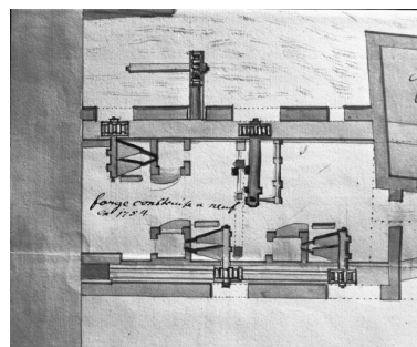
Plan de la forge de Chagey [détail]. Phot. Yves Sancey IVR43_19907000175X
