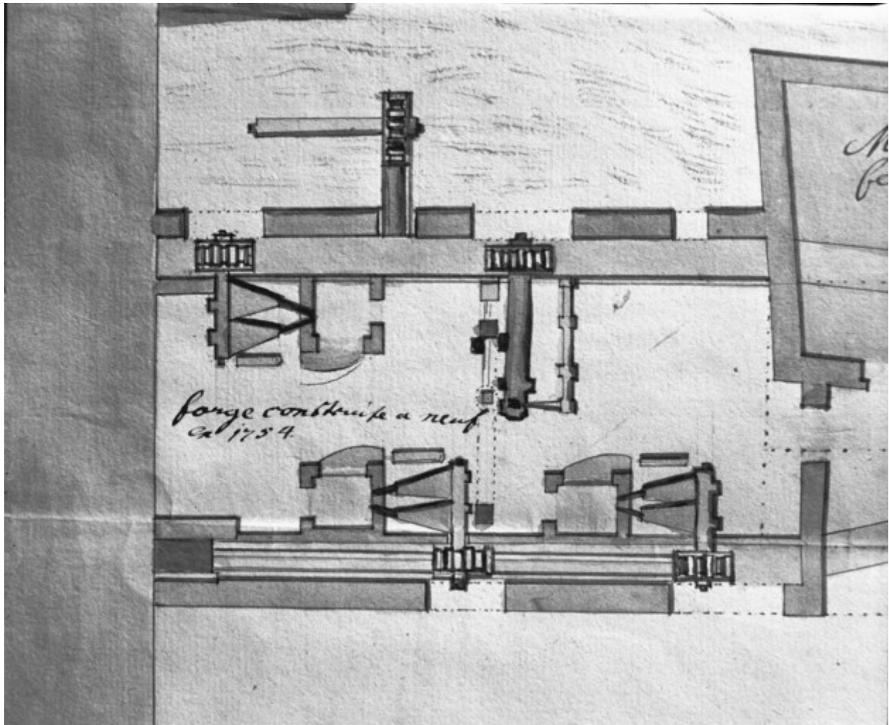
Plan de la forge de Chagey [détail].
