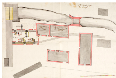
[Plan de la forge de Chagey : halle pour le charbon, 1754 (?)]. Phot. Jérôme Mongreville IVR43_20077000039NUCA
