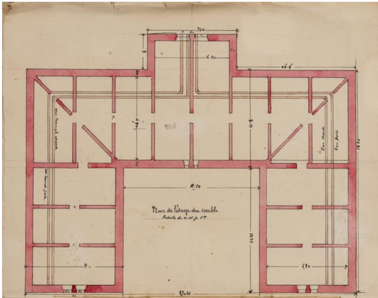
Plan des combles (1895).
