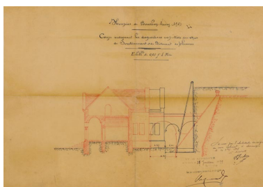
Coupe montrant la modification du projet initial (décalage de l'édifice vers le nord). Repro. Pierre-Marie Barbe- Richaud, Autr. François Dulac IVR26_20217100365NUC4A
