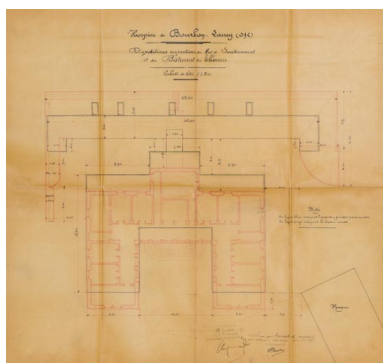
Plan montrant la modification du projet initial (décalage de l'édifice vers le nord). Repro. Pierre-Marie Barbe- Richaud, Autr. François Dulac IVR26_20217100364NUC2A
