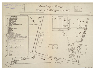
Plan de l'usine de Pontarlier, 1920. Phot. Jérôme Mongreville IVR43_20182500155NUC4A
