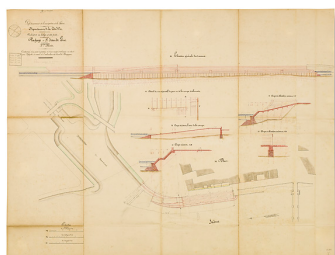
Construction d'un port à gradins et d'une rampe d'abreuvoir au droit du quai Lafayette en amont de l'embouchure du Canal de Bourgogne. Elévation, plan et coupe. Phot. Thierry Kuntz IVR26_20207100010NUC4A
