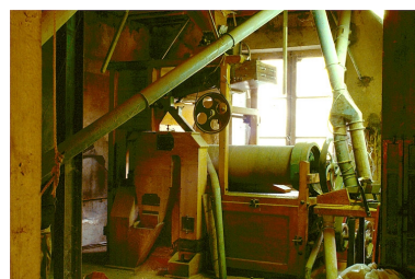
Minoterie (H), rez-de-chaussée : trieur à grains Lhuillier. Phot. Laurent Poupard IVR43_19883900522ZA
