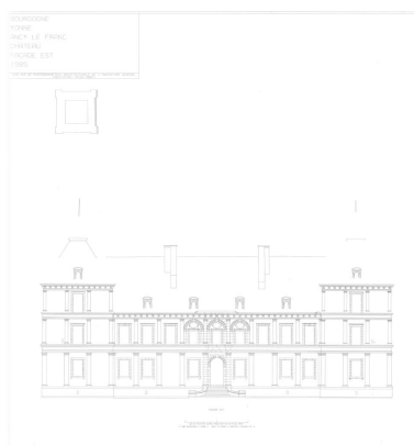
Façade est, restitution photogrammétrique. IVR26_20128900001A1YY
