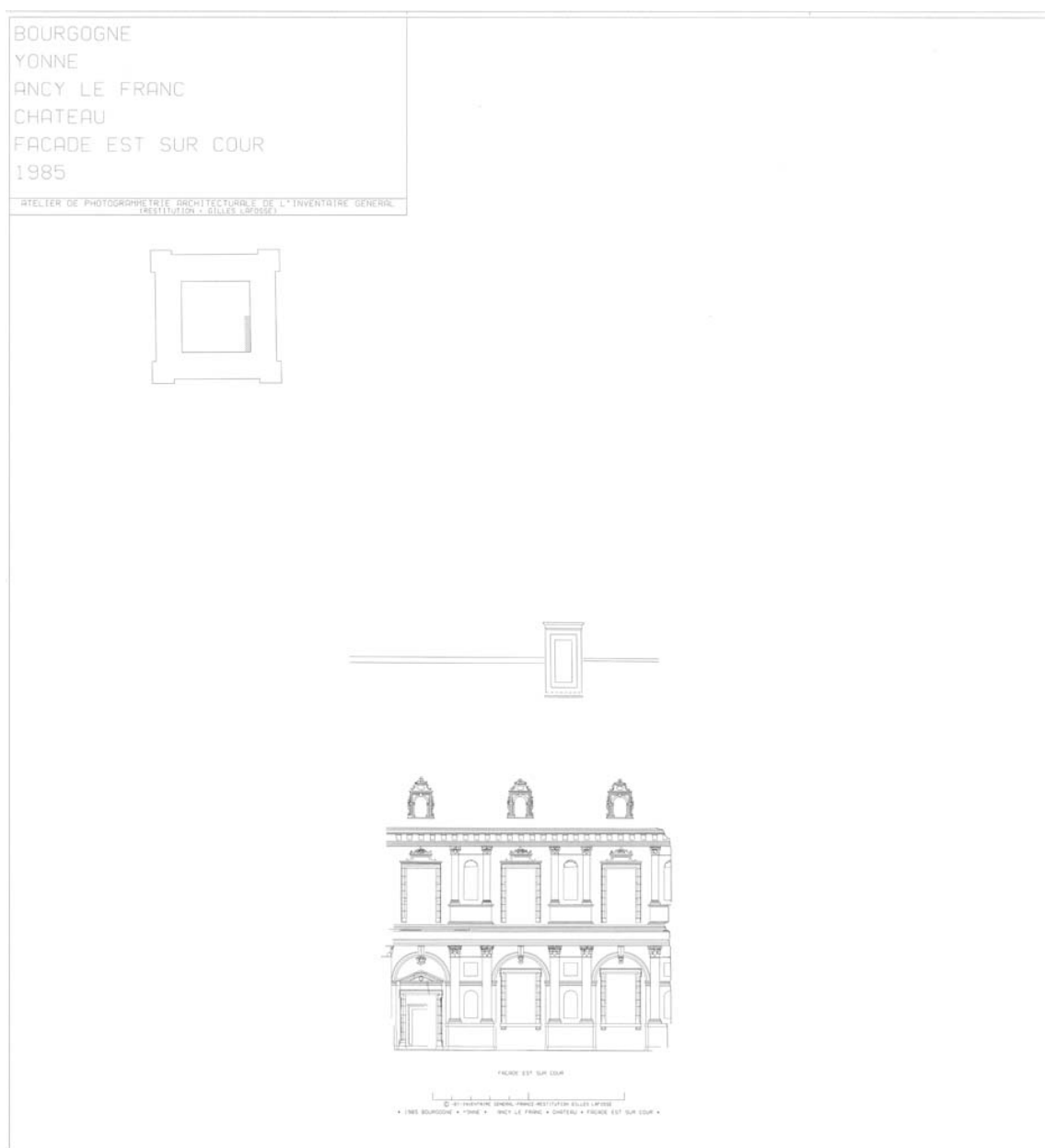
Façade est sur cour, restitution photogrammétrique.
