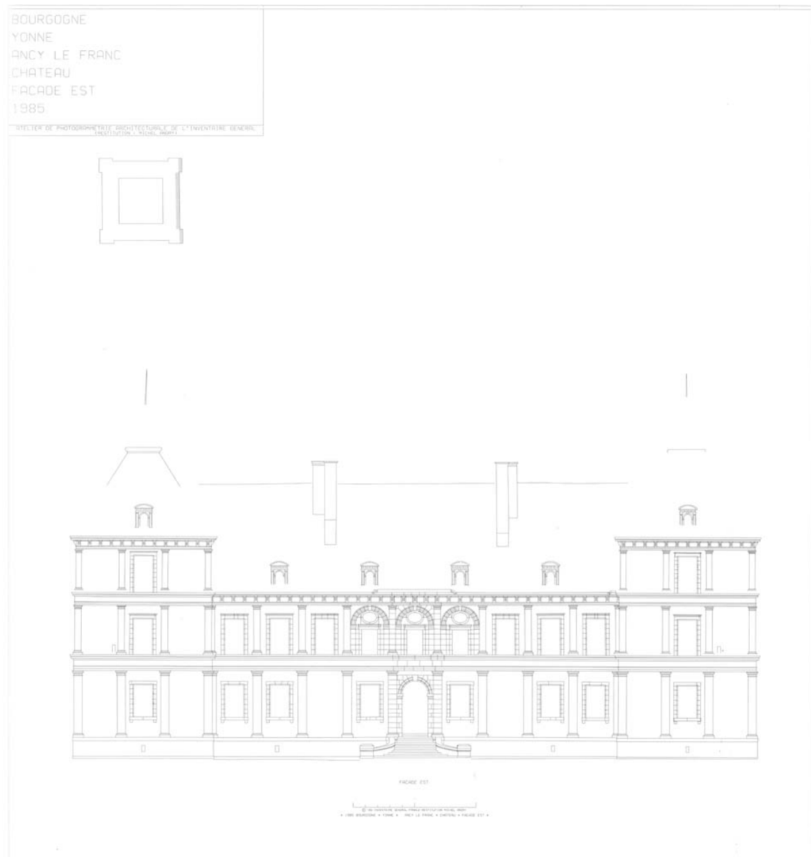
Façade est, restitution photogrammétrique.
