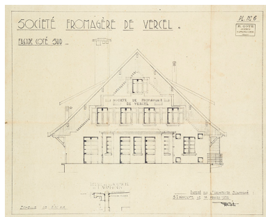
Société fromagère de Vercel. Façade côté sud, 1938. Phot. Jérôme Mongreville IVR43_20152500570NUC4A
