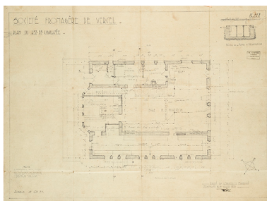
Société fromagère de Vercel. Plan du rez-de-chaussée, 1938. Phot. Jérôme Mongreville IVR43_20152500572NUC4A
