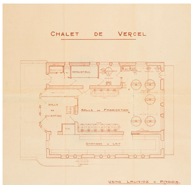
Chalet de Vercel. [Plan d'installation du matériel par la société Laurioz à Arbois], s.d. [1938] Phot. Jérôme Mongreville IVR43_20152500571NUC4A
