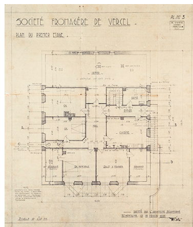
Société fromagère de Vercel. Plan du 1er étage, 1938. Phot. Jérôme Mongreville IVR43_20152500569NUC4A
