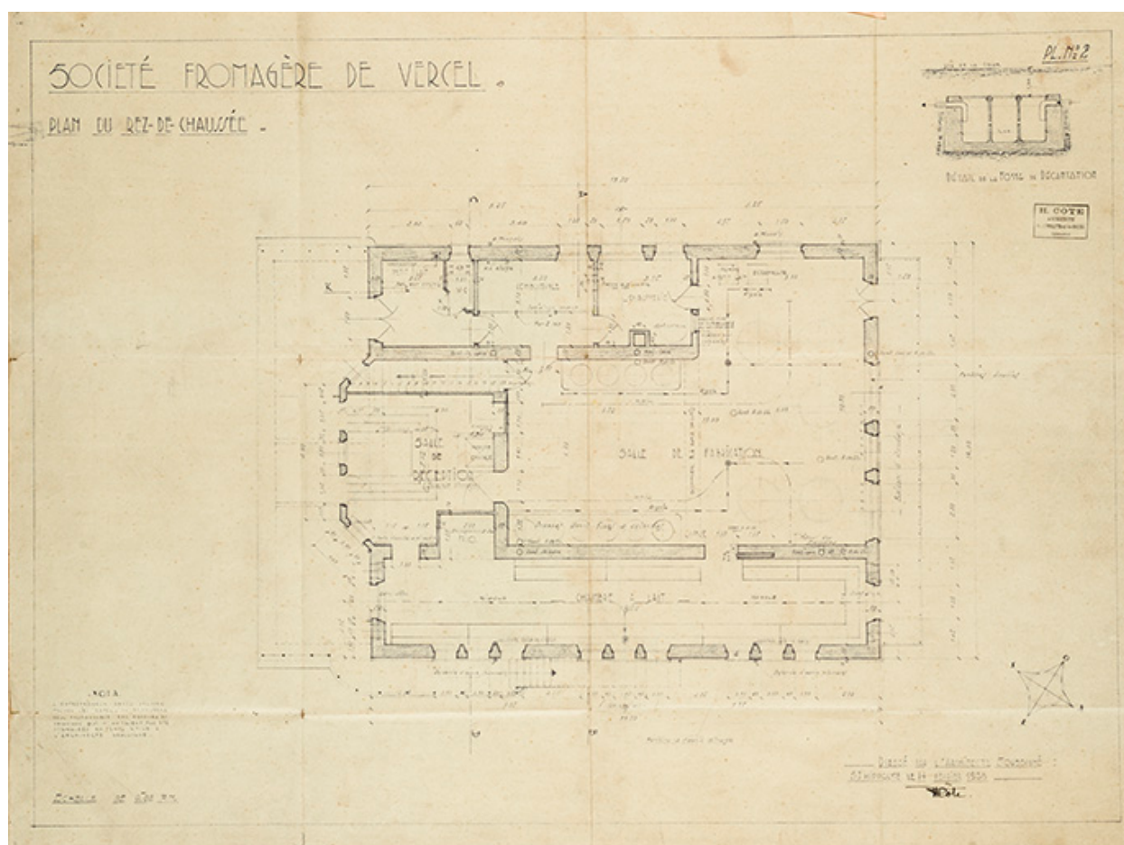
Société fromagère de Vercel. Plan du rez-de-chaussée, 1938.
