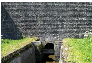
Sortie d'eau au pied du barrage pour la rigole d'alimentation du canal. Phot. Alain Morelière IVR26_20072106066NUC2A
