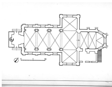
Plan au sol. Phot. Yves Sancey IVR43_19802500033V
