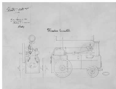
Machine locomobile [vue de face et de côté]. Phot. Jérôme Mongreville IVR43_20019000013V
