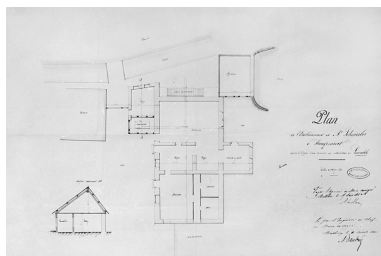
Plan de l'établissement de Mr Schmerber à Rougemont dressé à l'appui d'une demande en autorisation de locomobile. Phot. Jérôme Mongreville IVR43_20019000012V
