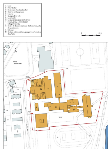
Plan-masse et de situation. Extrait du plan cadastral numérisé, section BO, échelle 1:1000. Dess. Mathias Papigny IVR43_20147000098NUDA
