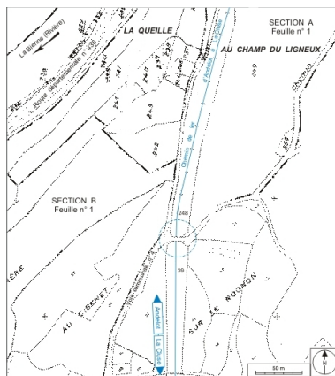
Plan-masse et de situation. Montage d'extraits du plan cadastral informatisé, 2006, sections A (1:2500) et B (1:1250), échelle 1:2000. Dess. André Céréza IVR43_20073900298NUDA
