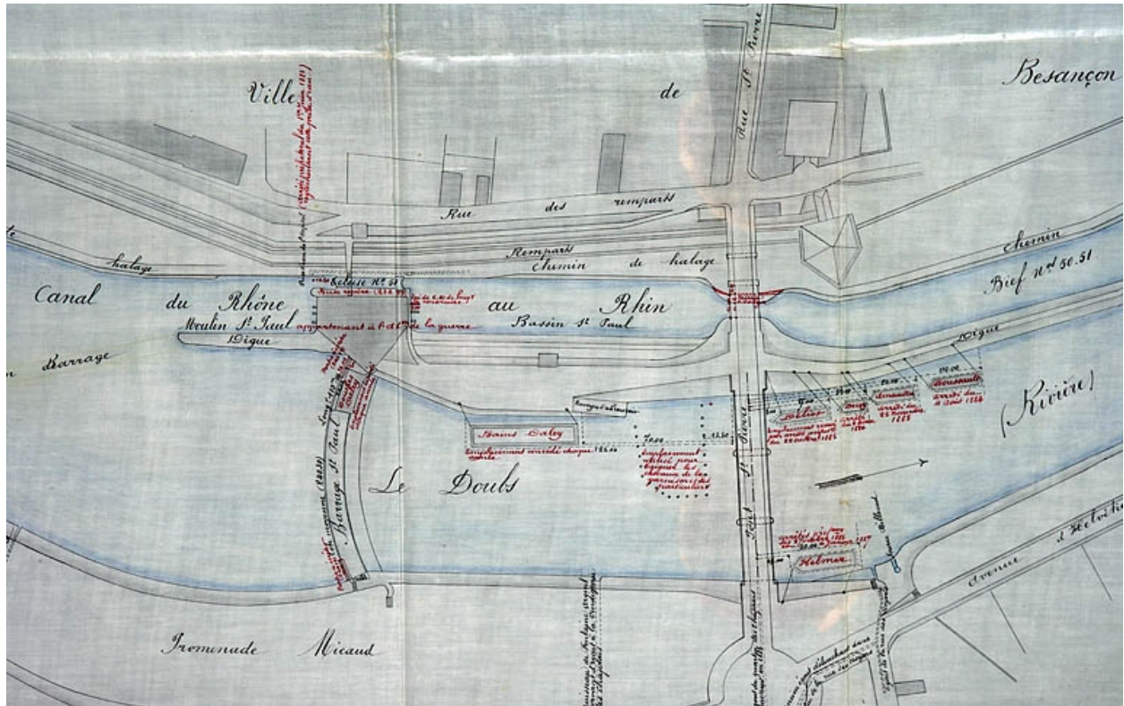
Règlement d'eau du moulin St Paul, appartenant à l'ad[ministrati]on de la Guerre. Plan des lieux [détail], 1887.
