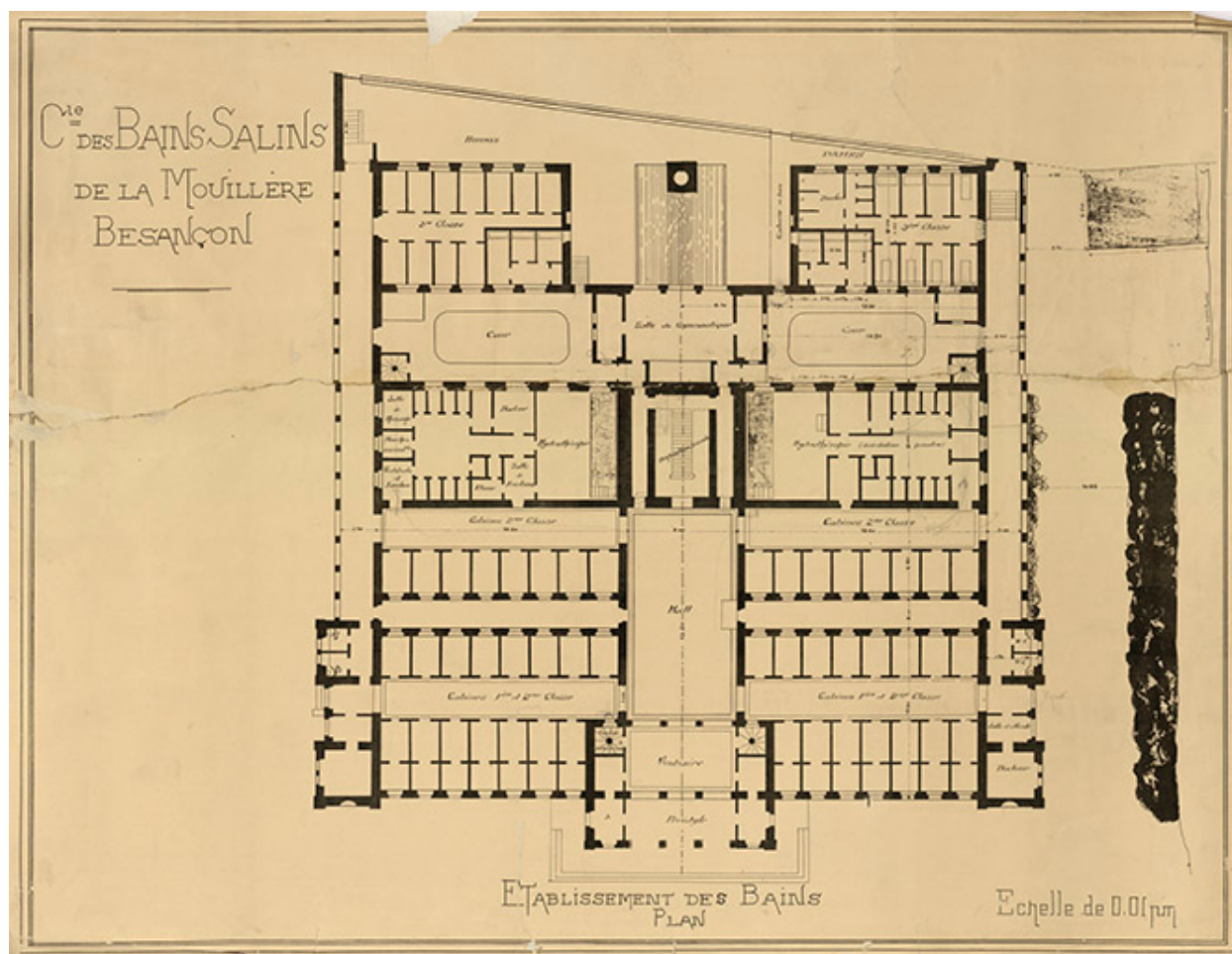
Plan du rez-de-chaussée (vers 1892).
