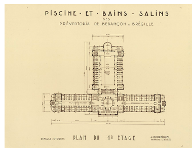
Projet de piscine et bains salins des Préventoria à Brégille, plan du premier étage (1935). Autr. Joseph Bourniquel IVR43_20232500573NUC4A
