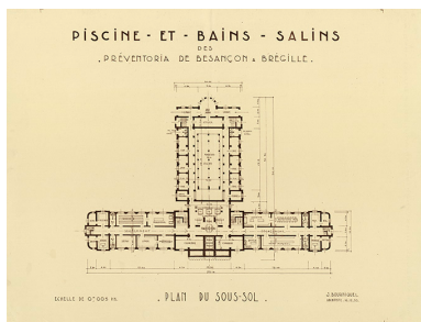
Projet de piscine et bains salins des Préventoria à Brégille, plan du sous-sol (1935). Autr. Joseph Bourniquel IVR43_20232500570NUC4A
