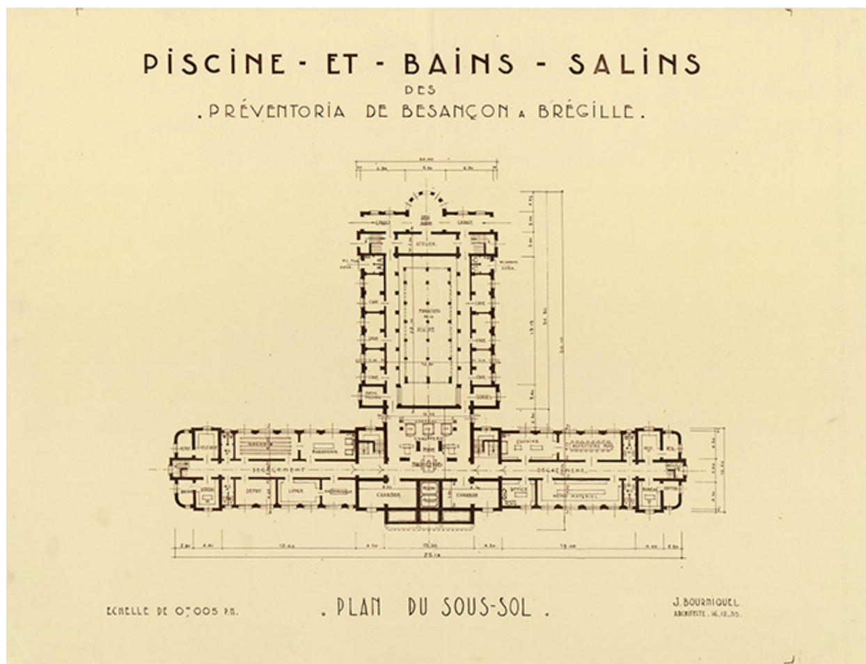
Projet de piscine et bains salins des Préventoria à Brégille, plan du sous-sol (1935).
