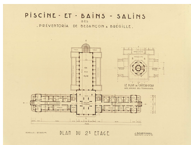
Projet de piscine et bains salins des Préventoria à Brégille, plan du deuxième étage (1935). Autr. Joseph Bourniquel IVR43_20232500574NUC4A
