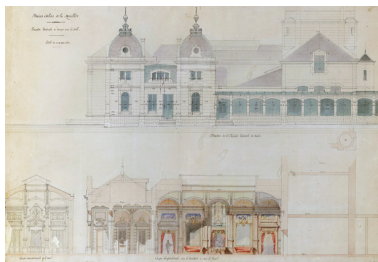
Façade latérale, coupe transversale sur le hall, coupe longitudinale sur le vestibule et le hall, projet (vers 1891).
