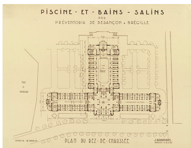
Projet de piscine et bains salins des Préventoria à Brégille, plan du rez-de-chaussée (1935). Autr. Joseph Bourniquel IVR43_20232500571NUC4A
