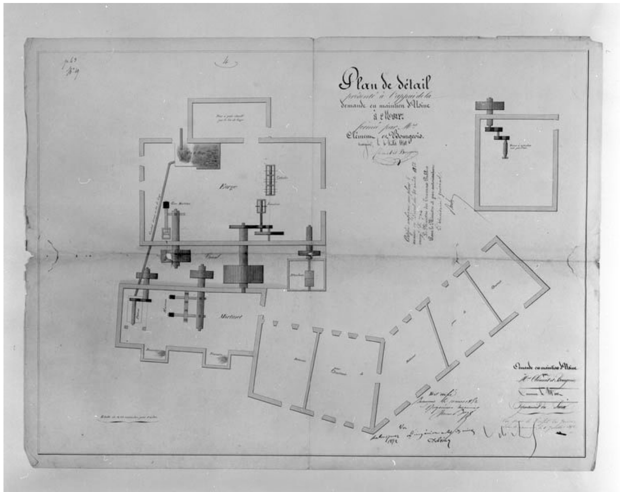
Plan de détail présenté à l'appui de la demande en maintien d'Usine à Morez formée par Mrs Clément et Bourgeois [...]. Dessin, 1840. Echelle 1:100.
