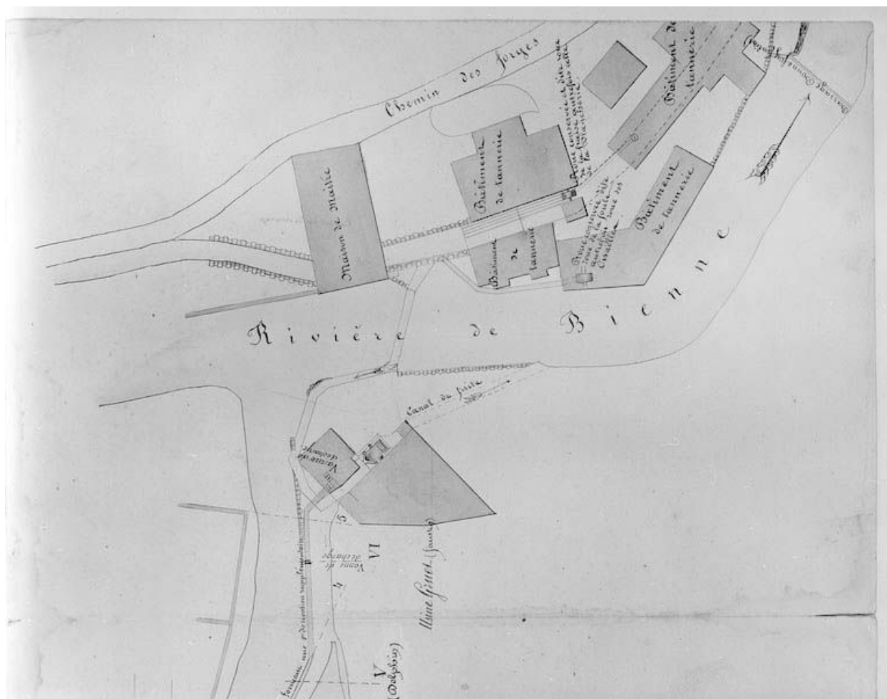
Réglement de l'usine Gruet Faustin. Plan [détail de la partie droite]. Dessin, 1859. Echelle 1:500.
