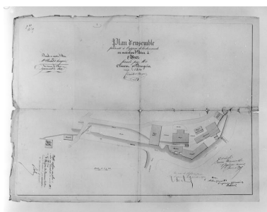
Plan d'ensemble présenté à l'appui de la demande en maintien d'Usine à Morez formée par Mrs Clément et Bourgeois [...]. Dessin, 1840. Echelle 1:500. Phot. Jérôme Mongreville, Autr. Paysant IVR43_19993900501V
