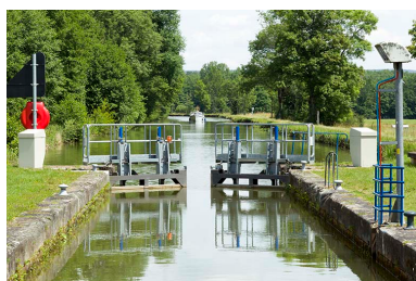
L'ouverture de portes vers l'amont à l'approche d'un bateau avalant. Phot. Sonia Dourlot IVR43_20157000949NUC2A
