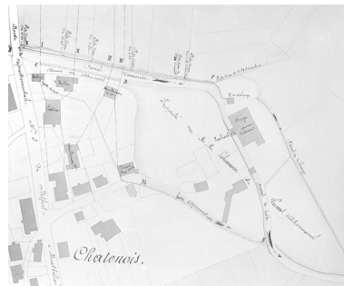
Plan des lieux [...] sur la demande des sieurs Vermot et Lehmann, tendant à réunir les 2 chutes en une seule. Phot. Jérôme Mongreville, Autr. Renault IVR43_20019000252X
