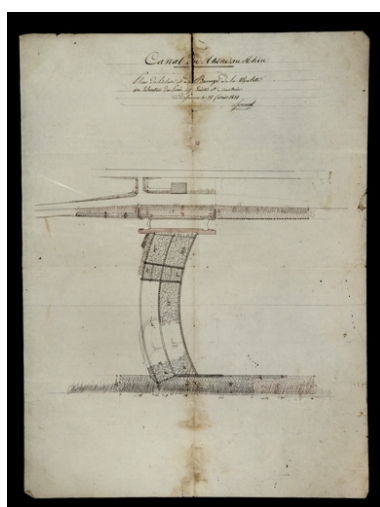
Plan de l'écluse et du barrage de la Malate avec l'élévation des perrés déjà exécutés et à construire, 1831. Phot. Yves Sancey, Autr. Formet (?) IVR43_20062500366NUCA
