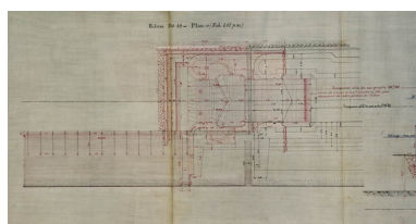
Allongement des écluses n° 49 et 52. Ecluse n° 49 de la Malate. Plan et coupes, 1883. Phot. Yves Sancey, Phot. Paul Schoendoerffer IVR43_20062500351NUCA
