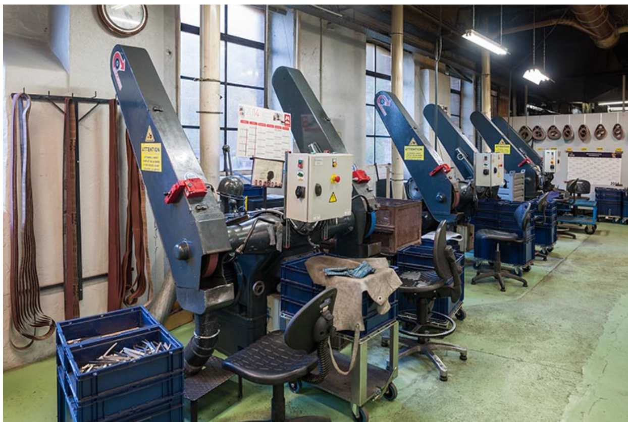
Postes de polissage.
