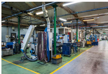
Atelier d'usinage. Vue de trois quarts. Phot. Jérôme Mongreville IVR43_20142501622NUC4A
