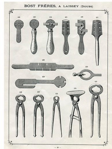
[Tourne-à-gauche, tenailles, etc.], catalogue Bost Frères, 1907. Phot. Jérôme Mongreville IVR43_20142501681NUC4A
