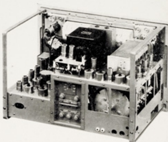
Le chassis du 2 e changeur de fréquence est représenté non muni de son capot de blindage.
