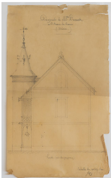
Projet de transformation, élévation du mur pignon nord-est. Phot. Pierre-Marie Barbe- Richaud, Autr. Adolphe Bouveault IVR26_20205800116NUC4A
