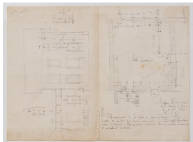
Plan de la salle à manger et élévation du pavillon avant l'intervention d'Adolphe Bouveault. Phot. Pierre-Marie Barbe- Richaud, Autr. Adolphe Bouveault IVR26_20205800118NUC4A
