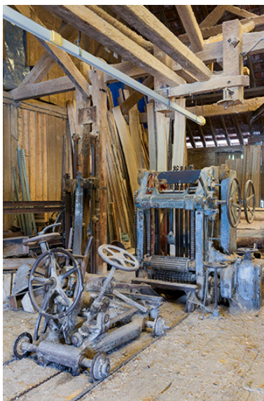
Châssis multilames et son chariot. Vue de trois quarts. Phot. Jérôme Mongreville IVR43_20162500436NUC4A
