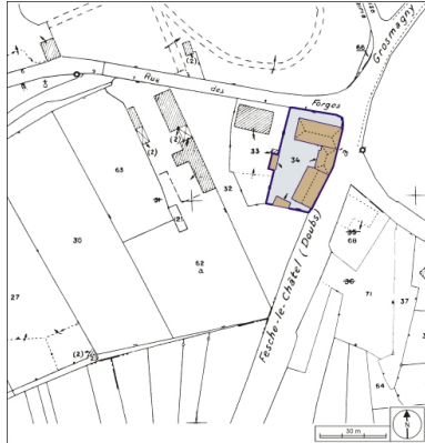
Plan-masse et de situation. Extrait du plan cadastral, 1984, section B, 1:1000. Dess. André Céréza IVR43_20039000038NUDA
