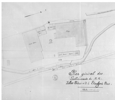
Plan général des établissements de MM. Zeller frères et Cie à Etueffont-Bas. Phot. Jérôme Mongreville IVR43_20019000004V
