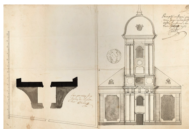
Faivre. Plan et élévation du clocher de l'église paroissiale Saint- Martin de Scey-sur-Saône. 1755. Phot. Jérôme Mongreville, Autr. Hugues Faivre IVR43_20197000001NUC4A
