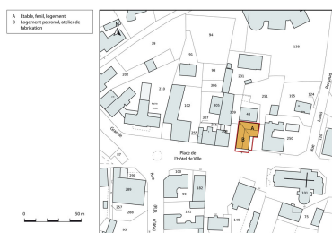
Plan-masse et de situation. Extrait du plan cadastral, 2015, section AC. Dess. Mathias Papigny IVR43_20152500676NUDA
