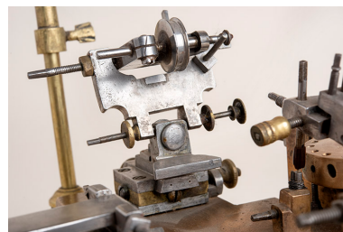
Support de la meule en saphir (à droite), avec sa poulie motrice. Phot. Sonia Dourlot IVR43_20192500441NUC4A
