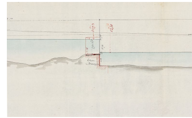
La Seille, profil en long. Daté de 1815. Détail de l'écluse de Branges. (Archives VNF-direction territoriale Centre-Bourgogne ; subdivision de Montceau-les-Mines) Phot. Jean-Luc Duthu IVR26_20107100251NUC2A
