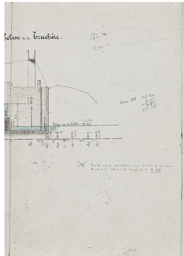
"Nivellement de la Seille, profils", par l'ingénieur Fournier, vers 1850. Croquis non datés des ponceaux et aqueducs du chemin de halage. Extrait : Ecluse de La Truchère, km 0 à 1. (Archives VNF-direction territoriale Centre-Bourgogne ; subdivision de Montceau-les-Mines) Phot. Pierre-Marie Barbe- Richaud, Autr. Fournier IVR26_20107100583NUC2A
