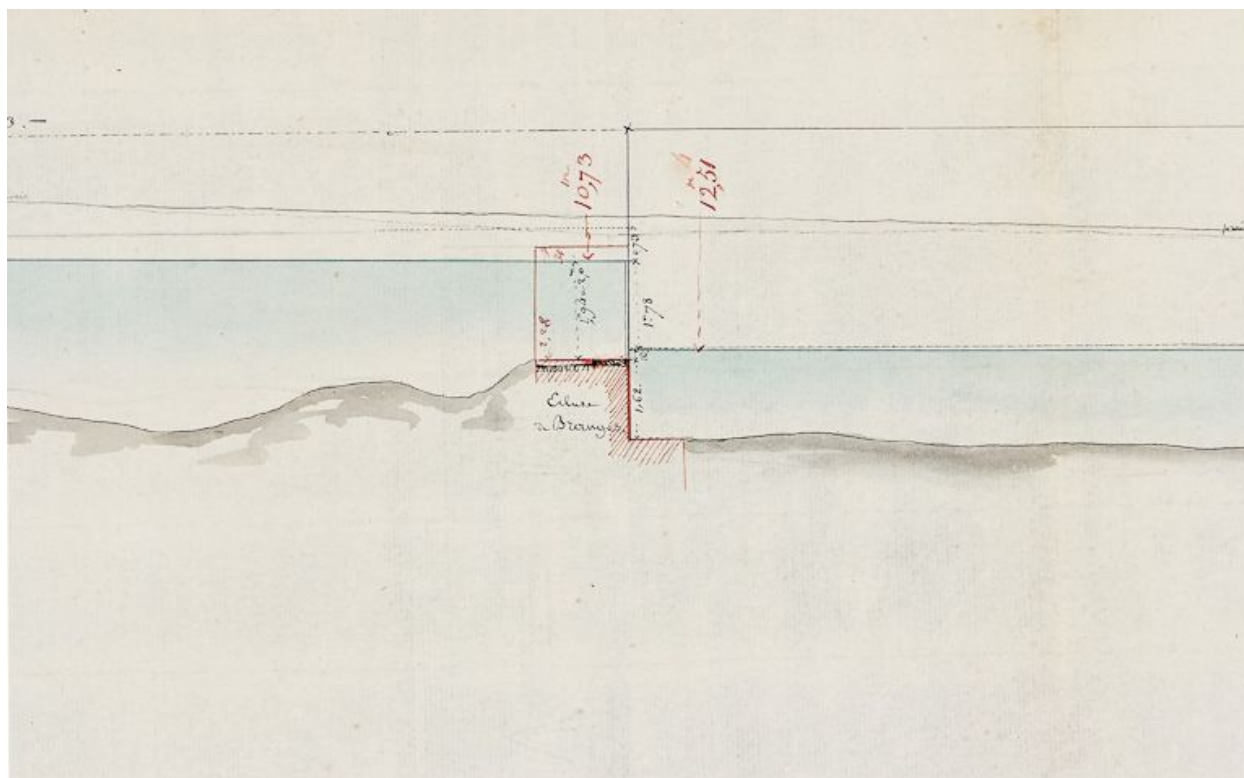
La Seille, profil en long. Daté de 1815. Détail de l'écluse de Branges. (Archives VNF-direction territoriale Centre-Bourgogne ; subdivision de Montceau-les-Mines)
