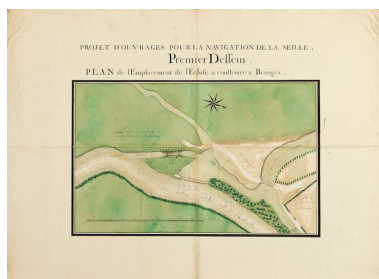
Projet d'ouvrages pour la navigation de la Seille. Premier dessin. Plan de l'emplacement de l'écluse à construire à Branges. Ce sont probablement les plans d'origine (1784) avec détail d'implantation des écluses. (Archives VNF-direction territoriale Centre-Bourgogne ; subdivision de Montceau-les-Mines) Phot. Jean-Luc Duthu IVR26_20107100260NUC4A
