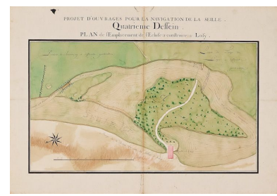
Projet d'ouvrage pour la navigation de la Seille. Quatrième dessin. Plan de l'emplacement de l'écluse à construire à Loisy. Il s'agit probablement d'un plan d'avant 1784. (Archives VNF-direction territoriale Centre-Bourgogne ; subdivision de Montceau-les-Mines) Phot. Jean-Luc Duthu IVR26_20107100235NUC2A
