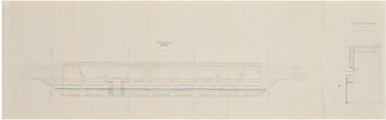
Construction de l'usine-moulin de La Truchère. Plan de l'usine et du barrage, élévation et coupe. Détail. (Archives VNF-direction territoriale Centre-Bourgogne ; subdivision de Montceau-les-Mines)
