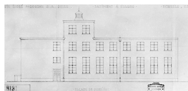
Fil Isolé Moderne S.A. Delle - Bâtiment à étages. Façade de derrière - R 131. Phot. Jérôme Mongreville, Phot. Buhlmann, Phot. Schibler IVR43_20019000008V
