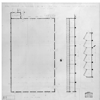
Fil Isolé Moderne S.A. Delle - Nouveau bâtiment de shed - R 11 [Coupes et plan au sol]. Phot. Jérôme Mongreville, Phot. Buhlmann, Phot. Schibler IVR43_20019000014V
