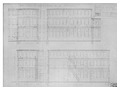
Fil Isolé Moderne S.A. Delle - Bâtiment à étages. Agrandissement 1929. Coupes - T 3.1. Phot. Jérôme Mongreville, Phot. Preiswerk et Cie IVR43_20019000021V
