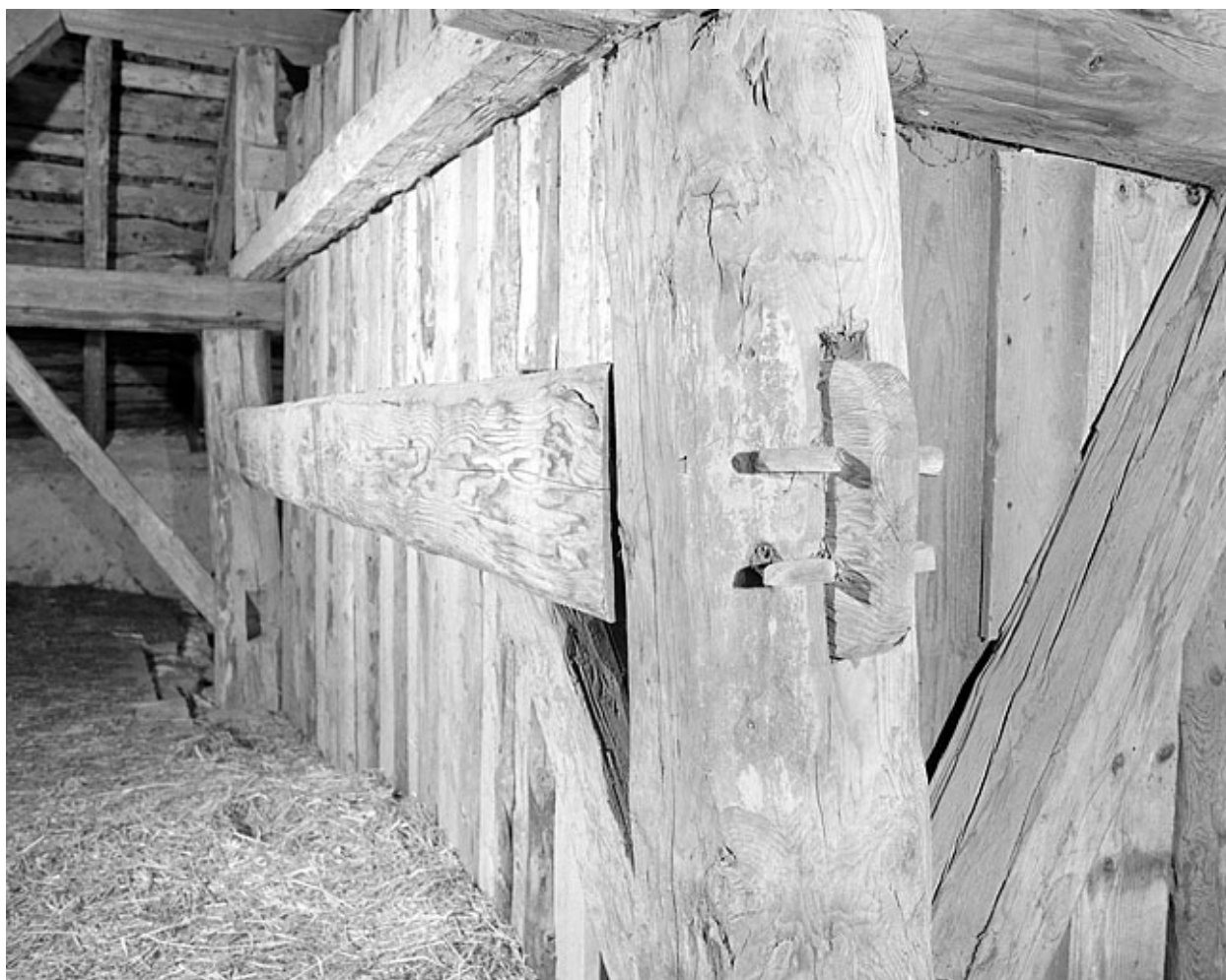
Assemblage de la charpente dans les combles.
