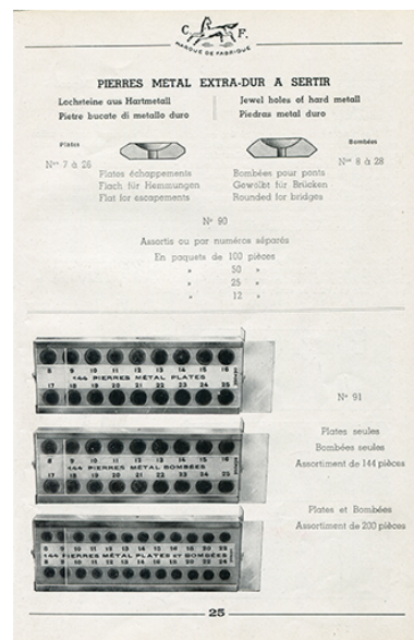
[Exemples de production de la société Cheval Frères :] Pierre métal extra-dur à sertir, 1950. Autr. auteur inconnu IVR43_20182501483NUC2A
