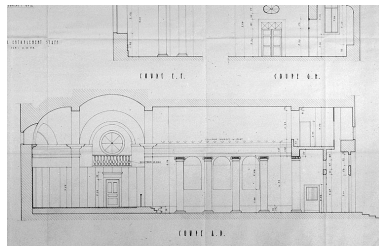
Coupe longitudinale.
