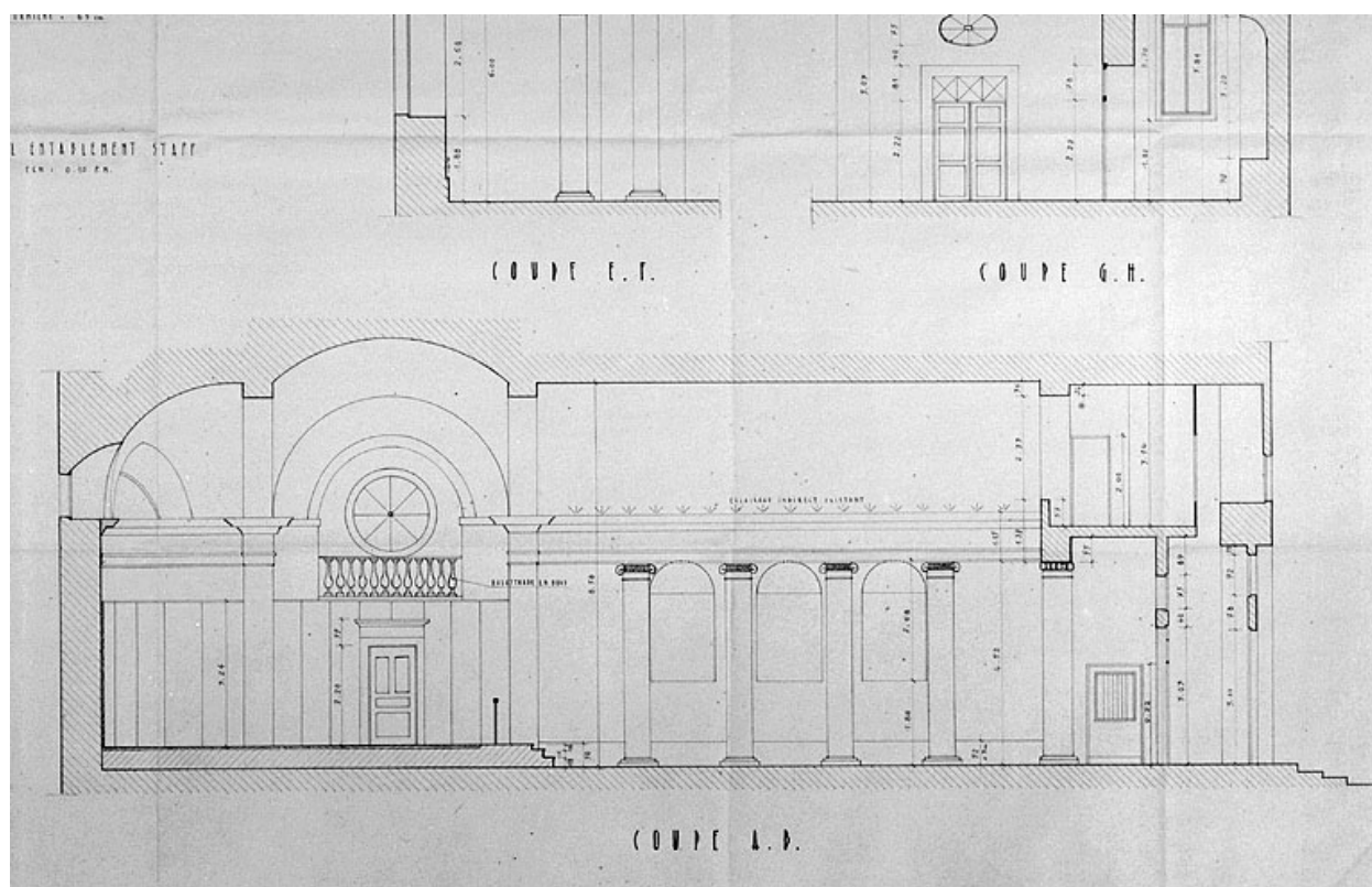
Coupe longitudinale.
