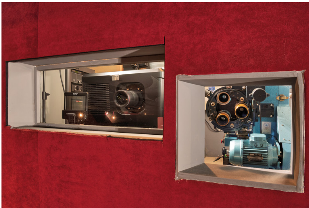
Salle 1 : fenêtres de projection. Projecteurs numérique Barco (à gauche) et argentique Cinemeccanica (à droite).
