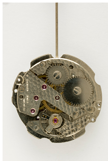
Mouvement France Ebauches FE 233-69-E-21 : face côté ponts. Phot. Sonia Dourlot IVR43_20162500761NUC4A
