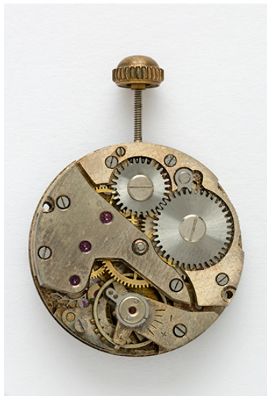
Mouvement Cupillard VC 233 : face côté ponts. Phot. Sonia Dourlot IVR43_20162500753NUC4A
