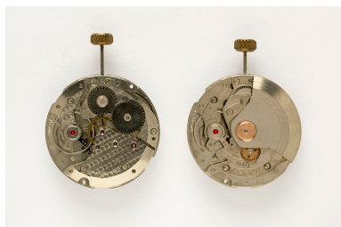
Mouvements France Ebauches FE 5601 (à gauche) et FE 5611 (à droite) : face côté ponts. Phot. Sonia Dourlot IVR43_20162500747NUC4A
