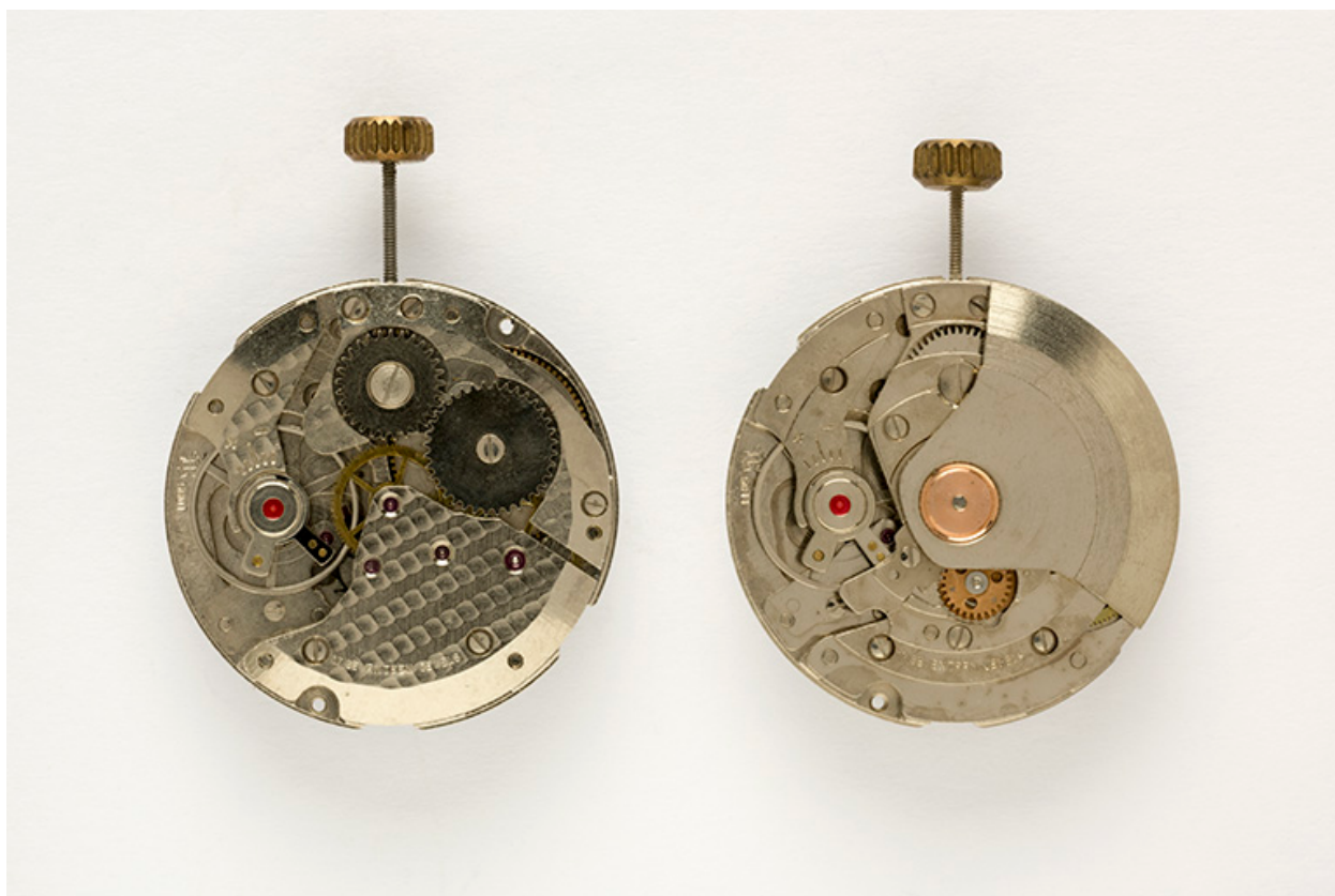
Mouvements France Ebauches FE 5601 (à gauche) et FE 5611 (à droite) : face côté ponts.
