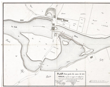
"Plan d'une partie du cours de la Seille, à joindre au rapport du soussigné en date de ce jour, sur la demande formée par M. de la Chapelle", par le conducteur faisant fonction d'ingénieur principal du 2e arrondissement Boulmicot, le 30 mai 1831. Il s'agit d'une demande du baron de la Chapelle pour conserver en leur état actuel les vannes et le déversoir de son moulin de Loisy. Avec le chemin de halage, les propriétés. (Archives VNF-direction territoriale Centre-Bourgogne ; subdivision de Montceau-les-Mines) Phot. Pierre-Marie Barbe-Richaud, Autr. Boulmicot IVR26_20107100674NUC4A
