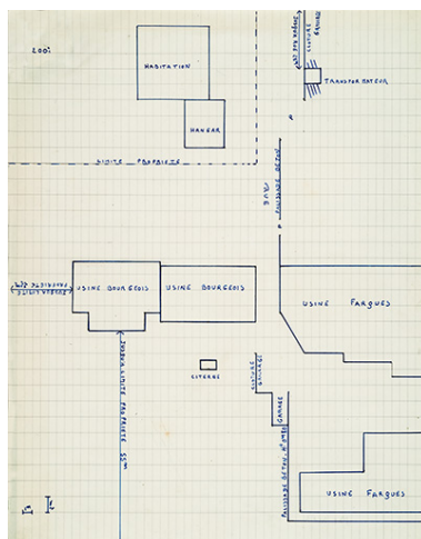
[Plan-masse et de situation de l'usine Étienne Bourgeois dressé à l'occasion de l'installation d'une citerne de gaz], [1964]. Phot. Jérôme Mongreville, Autr. auteur inconnu IVR43_20132500531NUC4A
