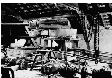
Système de distribution du mélange eau-sable : vue d'ensemble. Distributeur centrifuge surmonté d'un tamis en bois. Phot. Yves Sancey IVR43_19933900482ZA
