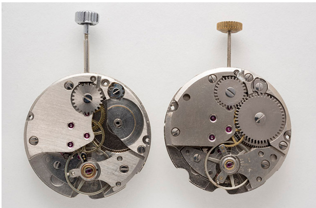
Deux mouvements de montre mécaniques France Ebauches FE 140-1 et 140-2A.
