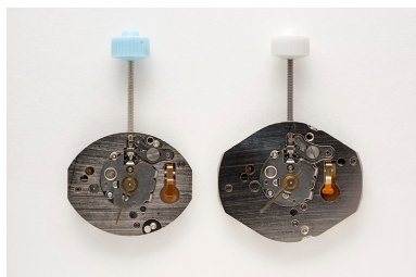
Deux mouvements de montre à quartz France Ebauches FE 5120 (à gauche) et 6120 (à droite). Phot. Sonia Dourlot IVR43_20152502573NUC4A
