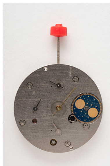
Mouvement de montre à quartz France Ebauches FE 11500. Phot. Sonia Dourlot IVR43_20152502570NUC4A
