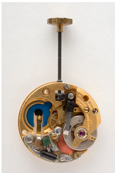
Mouvement de montre électromécanique Lip RE 50. Phot. Sonia Dourlot IVR43_20152502565NUC4A
