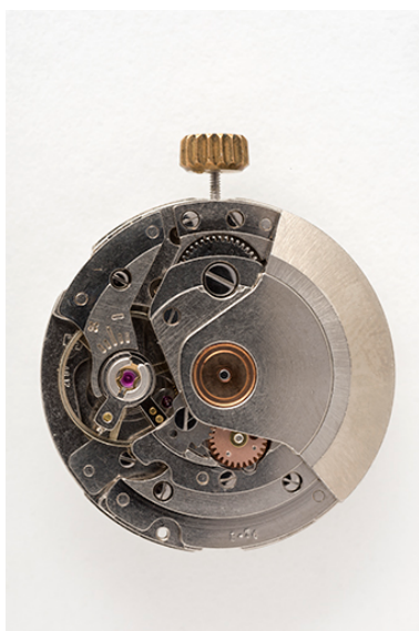
Mouvement de montre automatique France Ebauches FE 4612. Phot. Sonia Dourlot IVR43_20152502556NUC4A
