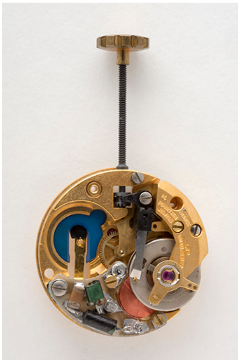
Mouvement de montre électromécanique Lip RE 50.
