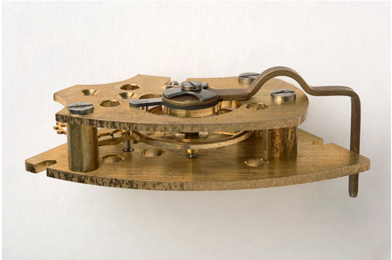
Echappement à chevilles et porte-échappement de la société Jeambrun Appareillages.
