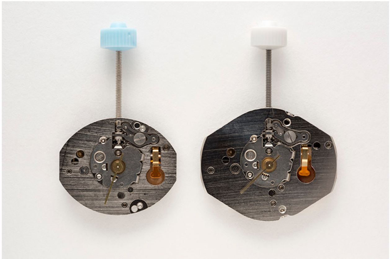
Deux mouvements de montre à quartz France Ebauches FE 5120 (à gauche) et 6120 (à droite).
