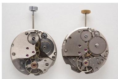
Deux mouvements de montre mécaniques France Ebauches FE 140-1 et 140-2A. Phot. Sonia Dourlot IVR43_20152502548NUC4A
