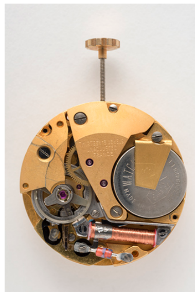
Mouvement de montre électromécanique Lip R 148. Phot. Sonia Dourlot IVR43_20152502569NUC4A
