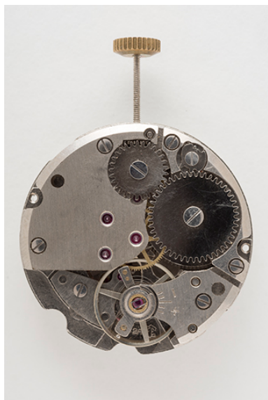
Mouvement FE 140-2A, vu côté pont. Phot. Sonia Dourlot IVR43_20152502549NUC4A
