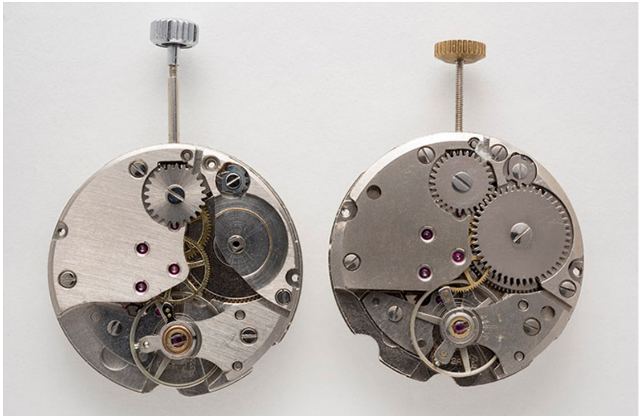
Les deux mouvements, vus côté pont : FE 140-1 à gauche, 140-2A à droite.
