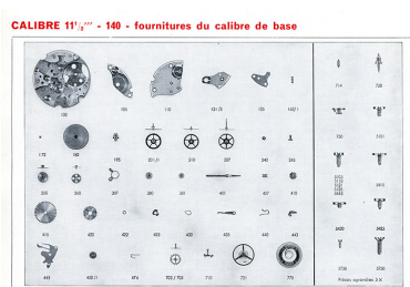
Calibre 11 1/2''' - 140 - fournitures du calibre de base, 1973.
