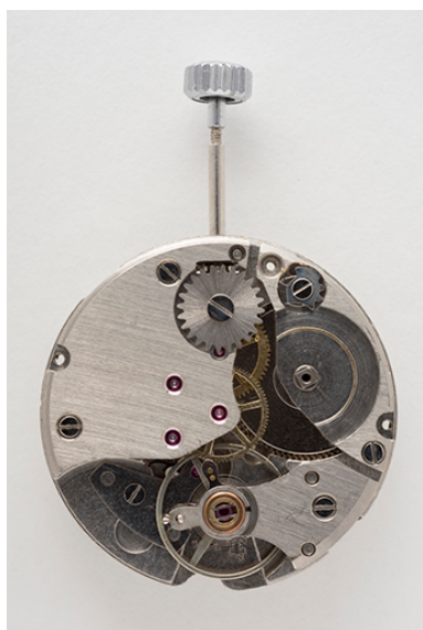
Mouvement FE 140-1, vu côté pont. Phot. Sonia Dourlot IVR43_20152502551NUC4A
