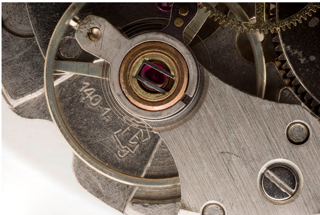
Mouvement FE 140-1 : logotype de la société France Ebauches et indication du modèle.
