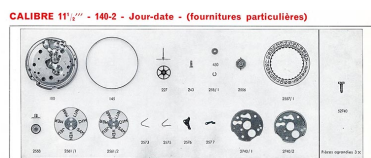
Calibre 11 1/2''' - 140-2 - Jour-date - (fournitures particulières), 1973.
