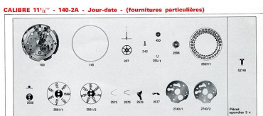
Calibre 11 1/2''' - 140-2A - Jour-date - (fournitures particulières), 1973.
