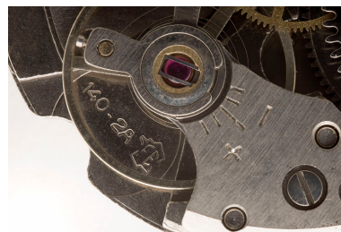
Mouvement FE 140-2A : logotype de la société France Ebauches et indication du modèle. Phot. Sonia Dourlot IVR43_20152502553NUC4A
