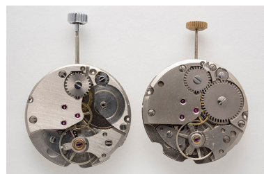
Les deux mouvements, vus côté pont : FE 140-1 à gauche, 140-2A à droite.
