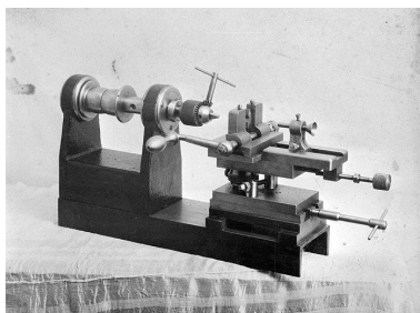
Exemple de machine à percer du constructeur mécanicien Lizon. Phot. Yves Sancey IVR43_20013900055X
