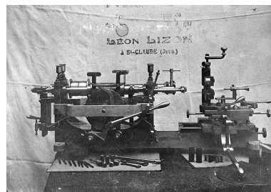
Exemple de "machine à monter universelle" du constructeur mécanicien Lizon. Phot. Yves Sancey IVR43_20013900056X
