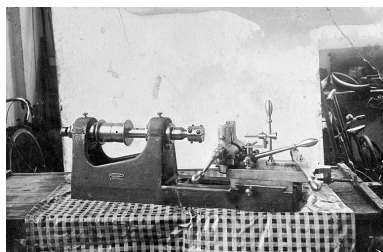
Exemple de machine à floquer du constructeur mécanicien Lizon. Phot. Yves Sancey IVR43_20013900054X
