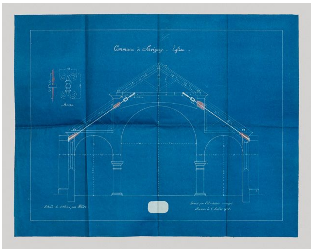
Coupe du projet de consolidation de l'église de Savigny-lès-Beaune. 6 juillet 1908. (Archives municipales, Savigny-lès-Beaune)
