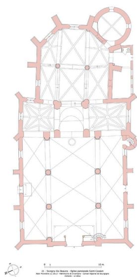
Plan de l'église. Dess. Alain Morelière IVR26_20132101080NUDA
