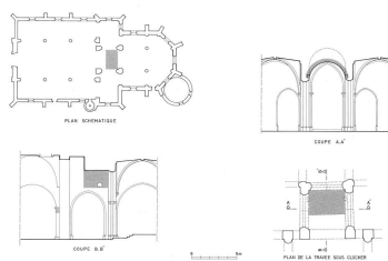
Plan, coupe et élévation schématiques de localisation des peintures murales.
