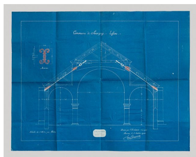
Coupe du projet de consolidation de l'église de Savigny-lès- Beaune. Louis Gagnerot - Architecte. 6 juillet 1908. (Archives municipales, Savigny-lès-Beaune) Phot. Pierre-Marie Barbe- Richaud, Autr. Louis Gagnerot IVR26_20172100003NUC2A
