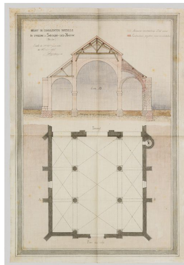
Projet de consolidation partielle de l'église de Savigny-lès- Beaune (Côte-d'Or)" : coupe et plan. Daté du 20 février 1874 et signé Deschamp. (Archives municipales, Savigny-lès-Beaune) Phot. Pierre-Marie Barbe- Richaud, Autr. Deschamp IVR26_20172100002NUC2A
