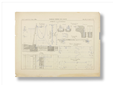
Barrage mobile de Poncey. Fermette et ses accessoires.1886. Phot. Thierry Kuntz IVR26_20172100145NUC4A
