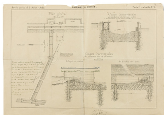
Barrage de Poncey. Plan général, coupes transversales du déversoir
