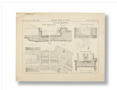
Barrage mobile de Poncey. Détail des maçonneries. 1886. Phot. Thierry Kuntz IVR26_20172100144NUC4A
