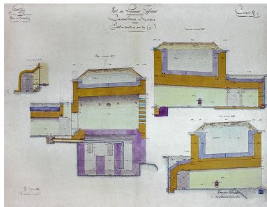
Caserne basse, vue en coupe. Phot. Schwartz IVR43_19802500810XE
