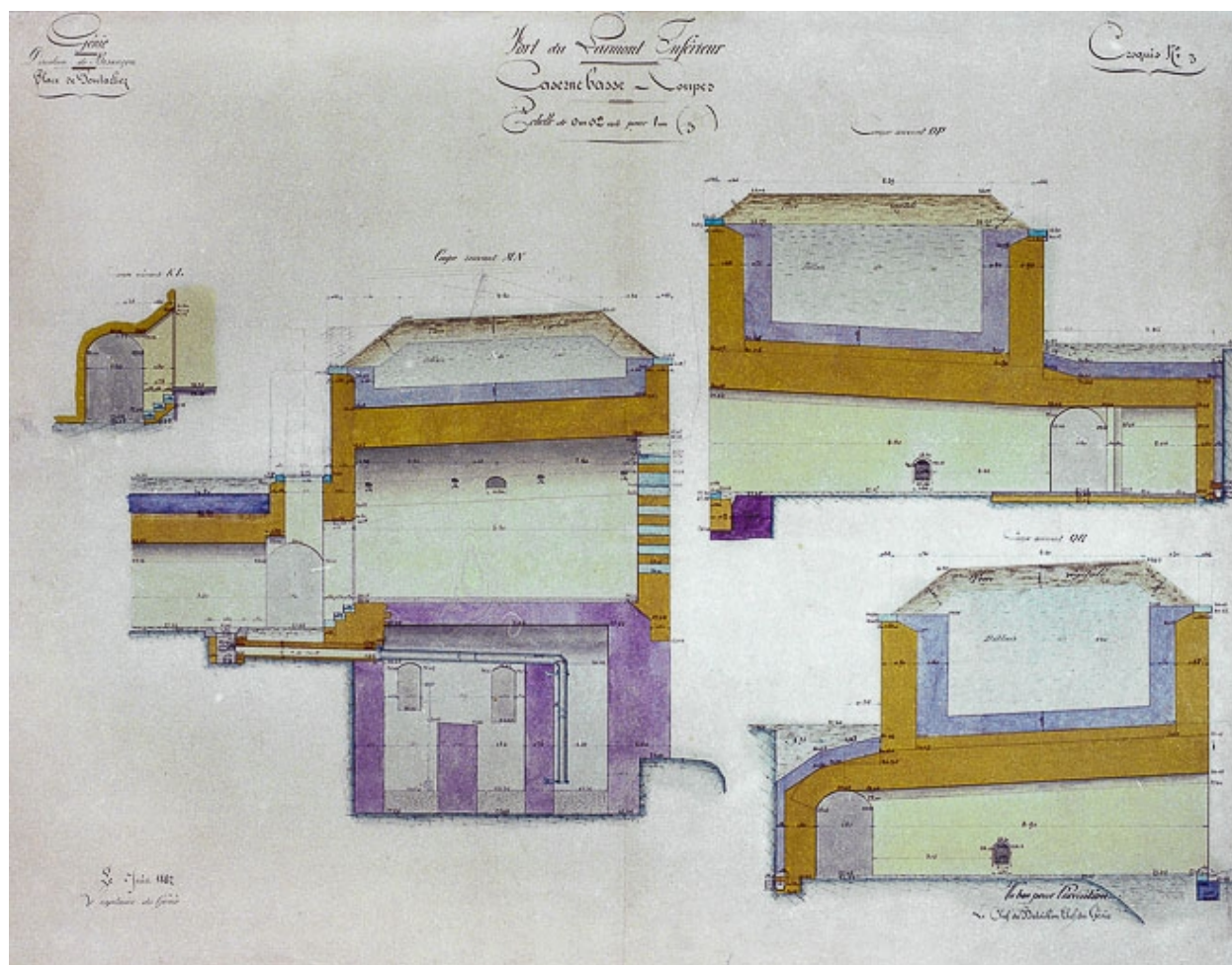
Caserne basse, vue en coupe.
