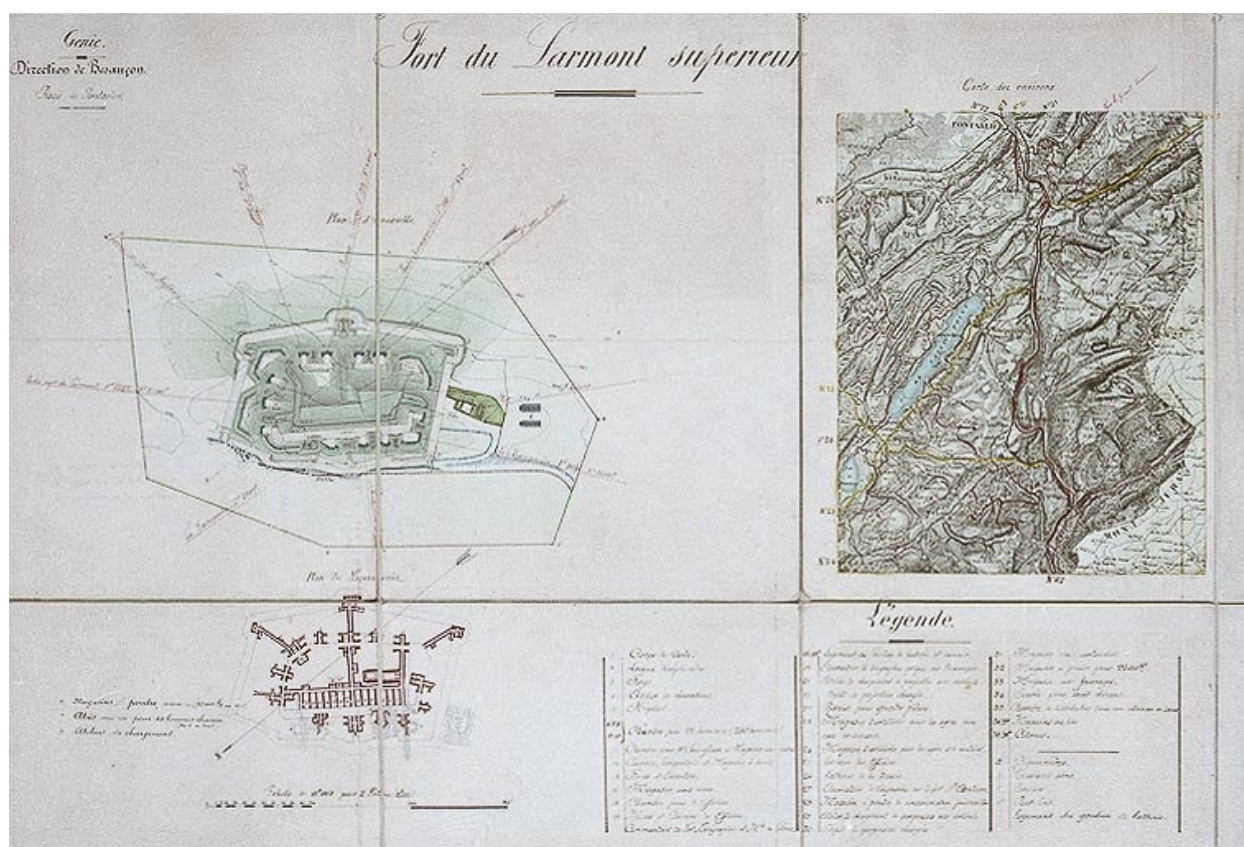
Plan du fort du Larmont supérieur, 1881. (article 8 section 2).
