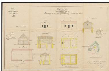
Bâtiment projeté pour corps de garde et logement du portier consigné à la porte de Comté. 1837. Autr. Thomassin IVR26_20232100140NUC4A
