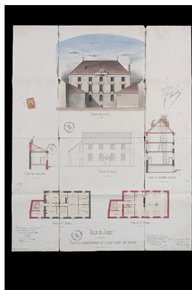
Projet d'agrandissement de l'école laïque de garçons [plans, élévation, coupes], 1879. Phot. Nicolas Waltefaugle IVR43_20257000206NUC4A
