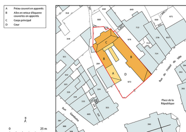
Plan-masse et de situation. Extrait du plan cadastral numérisé de la direction générale des finances publiques, 2025, 1/500. Dess. Aline Thomas IVR43_20257000045NUDA
